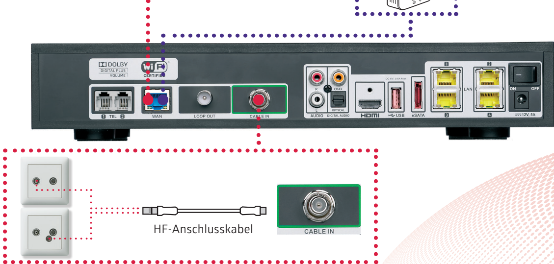
Anschluss an Quickline Box NACH Einführung der Zusatzbox
